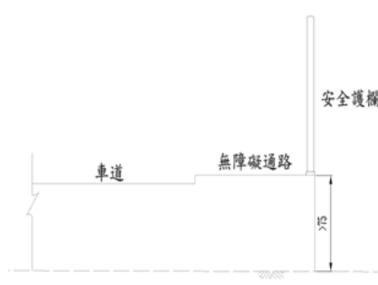
圖 14.1.1 無障礙通路設置防護緣示意圖
