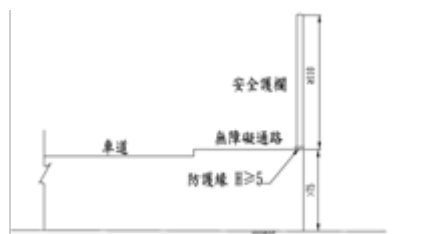
圖 14.1.1 無障礙通路設置防護緣示意圖
