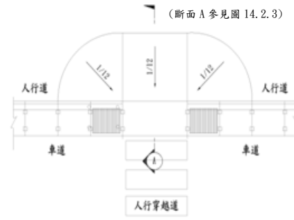
圖 14.2.1 路緣斜坡設計圖例(路段)
