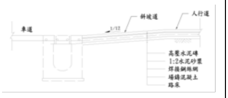
圖 14.2.3 路緣斜坡設計圖例(橫斷面)
